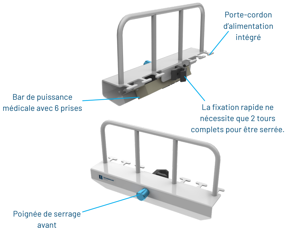
Porte-pompes à 4 appareils
